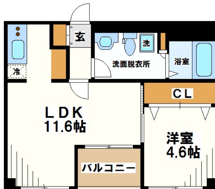
【間取り図】
